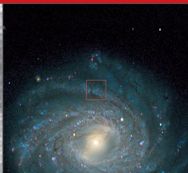
10 1 metri - Ecco la Via Lattea! È stato necessario percorrere 100 mila anni luce per vederla dall'esterno. Essa è composta da centinaia di miliardi di stelle, che si attraggono reciprocamente e che ruotano attorno al centro galattico, il Sole compie un giro in circa 300 milioni di anni.
