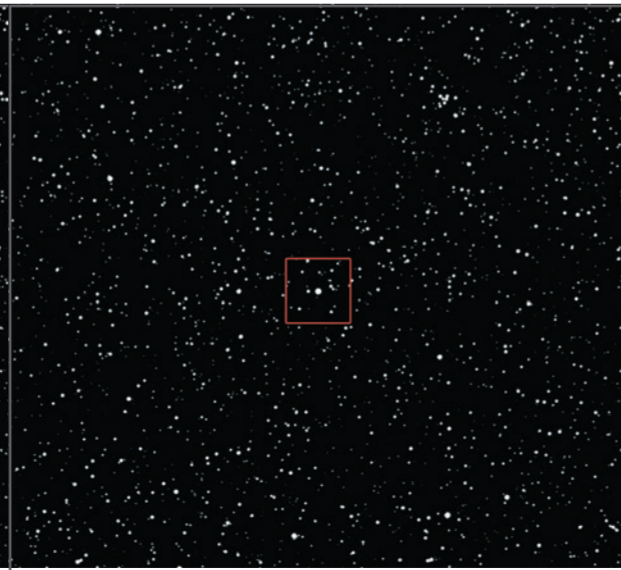
10 14 metri - A 1000 miliardi di chilometri di distanza dalla Terra ci troviamo ai confini del Sistema solare, immersi nella buia e fredda regione in cui orbitano le comete, che diventano visibili solo quando "cadono" verso le zone più vicine al Sole.
