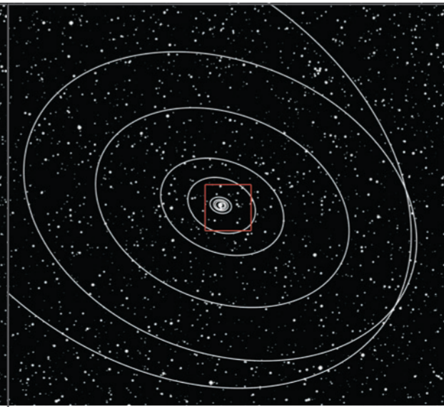
10 16 metri - A 10 miliardi di chilometri di distanza si vede tutta l'area percorsa dai pianeti del Sistema solare, sono evidenziate le orbite dei pianeti esterni (Giove, Saturno, Urano e Nettuno). Plutone, secondo la nuova classificazione dei corpi del Sistema solare, è il primo pianeta nano.
