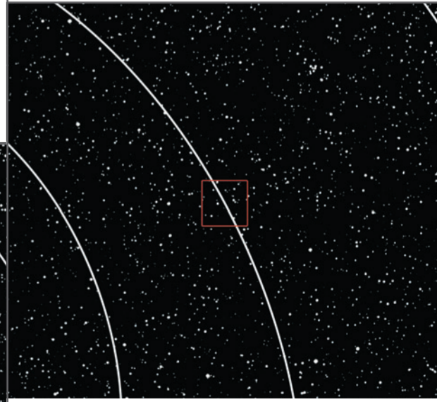
10 12 metri - Da 100 milioni di chilometri di distanza, vediamo parte delle orbite percorse dalla Terra e dai due pianeti ad essa più vicini, Venere all'interno (a sinistra) e Marte all'esterno (a destra dell'immagine).
