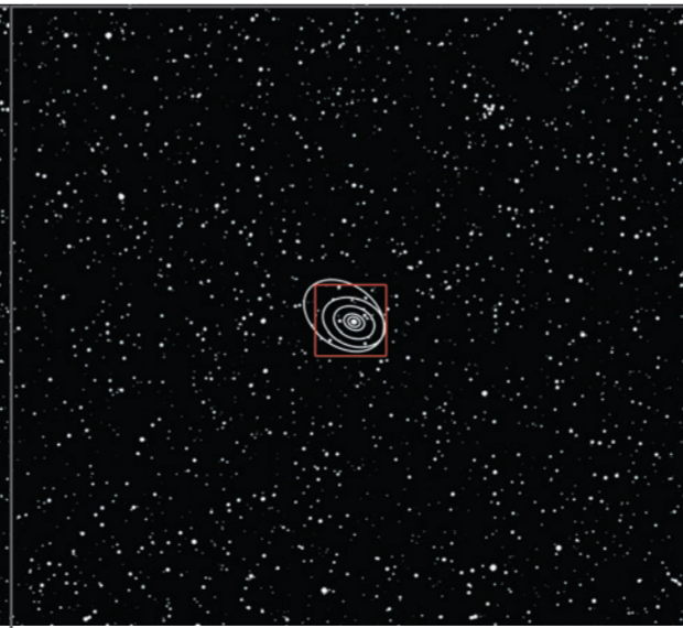
10 15 metri - Visti dall'esterno, a 100 miliardi di chilometri di distanza, i pianeti mostrano il loro carattere copernicano, con il Sole al centro del loro moto di rivoluzione, si muovono tutti in verso antiorario.
