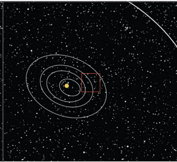
10 17 metri - Siamo a 1 miliardo di chilometri dal nostro Pianeta, pari a circa 7 Unità Astronomiche (1 U.A. = 149.597.870 km, distanza media della Terra dal Sole). Vediamo la nostra stella, il Sole, le orbite percorse dai pianeti interni (Mercurio, Venere, Terra e Marte) e parte dell'orbita di Giove.
